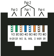
T568A
